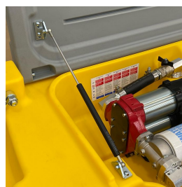
Pistoni a gas per apertura semi-automatica del coperchio e chiusura accompagnata
