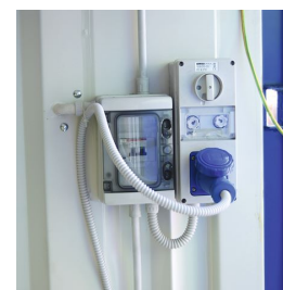
Impianto elettrico
