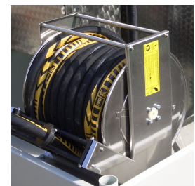
Avvolgitubo con guida
